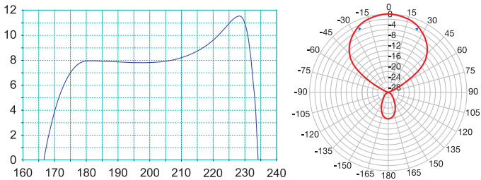
SIGMA V2 HD
